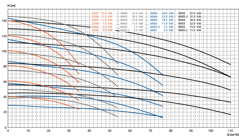
DeltaSolo D, système hydraulique tailles 25, 40, 60, 90, n ≈ 2900 rpm
