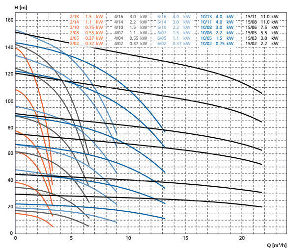
DeltaSolo D, système hydraulique tailles 2, 4, 6, 10, 15, n ≈ 2900 rpm
