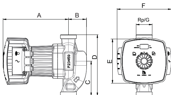
III. 5: Groupe motopompe à orifices filetés
