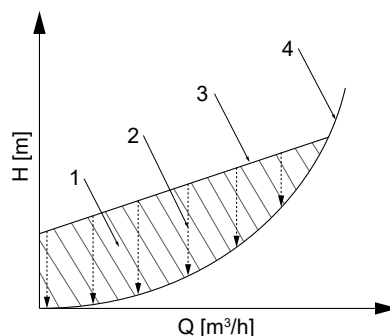
III. 3: Principe de la commande dynamique
