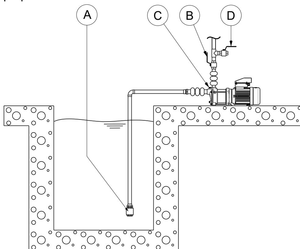
III. 7: Pompe en circuit ouvert, niveau de liquide situé en dessous de la pompe
