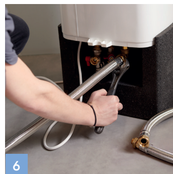
6 Raccorder les flexibles d'Easy Switch aux arrivées d'eau
